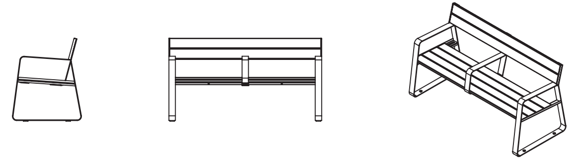
Largo: 1500 mm / Alto: 816 mm / Profundidad: 678 mm / Apoyabrazos: 3
