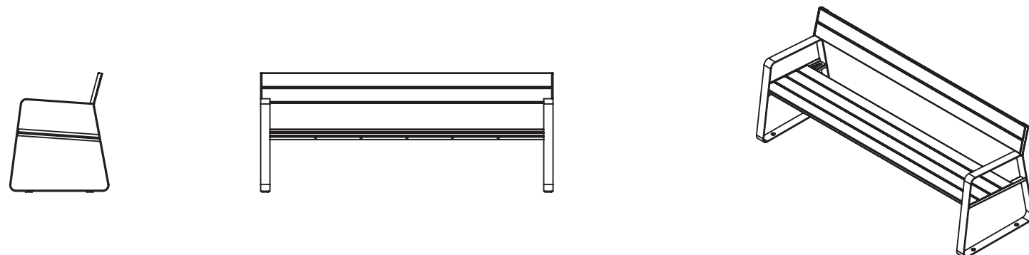
Largo: 2000 mm / Alto: 816 mm / Profundidad: 678 mm / Apoyabrazos: 2
