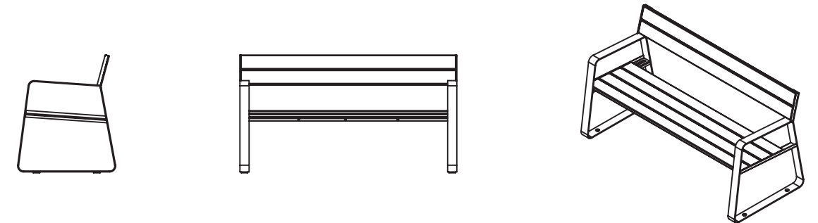
Largo: 1500 mm / Alto: 816 mm / Profundidad: 678 mm / Apoyabrazos: 2
